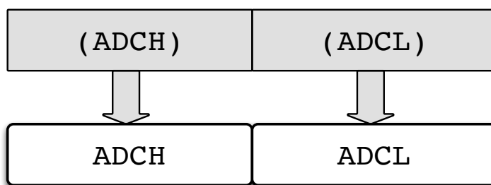
Figur 8.2.: Ett eventuellt nyare omvandlarresultat ligger färdigt att överföras till ADCH:ADCL. Överföringen sker inte förrän ADCH är läst för att inte kunna läsa resultat från två olika omvandlingar.
