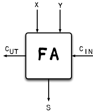
Figur 4.3.: Fulladderaren som vi minns den från digitaltekniken adderar tre inkommande bitar x , y och c_{in} till två bitar \{c_{ut}, s\} .
