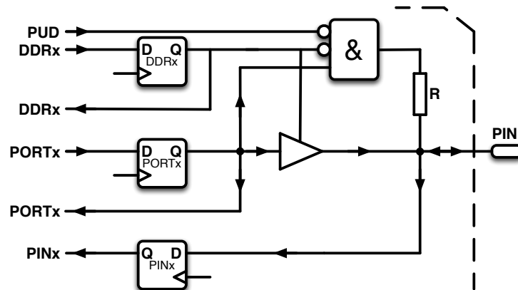
Figur 2.1.: Schemat visar en av åtta bitar i en port. Skrivning sker till PORTx och läsning från PINx . Biten konfigureras som in- eller utgång med datarikttningsregistret DDRx . Triangelsymbolen är tri-state-bufferten.
