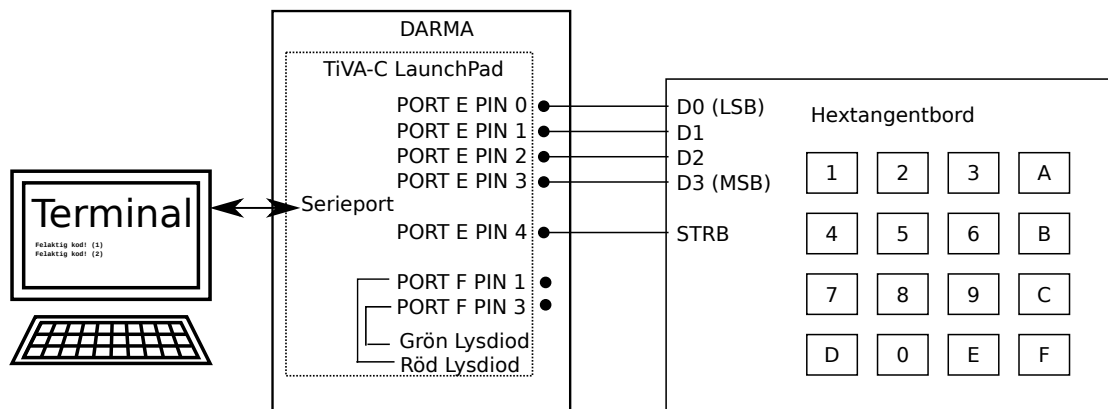
Figur 1: Labuppkopplingen
